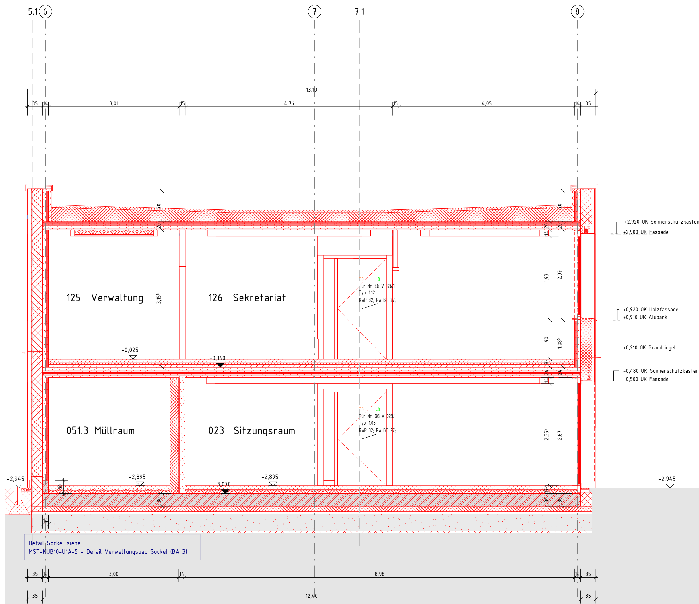
S11 - BA 3 M 1 : 50
