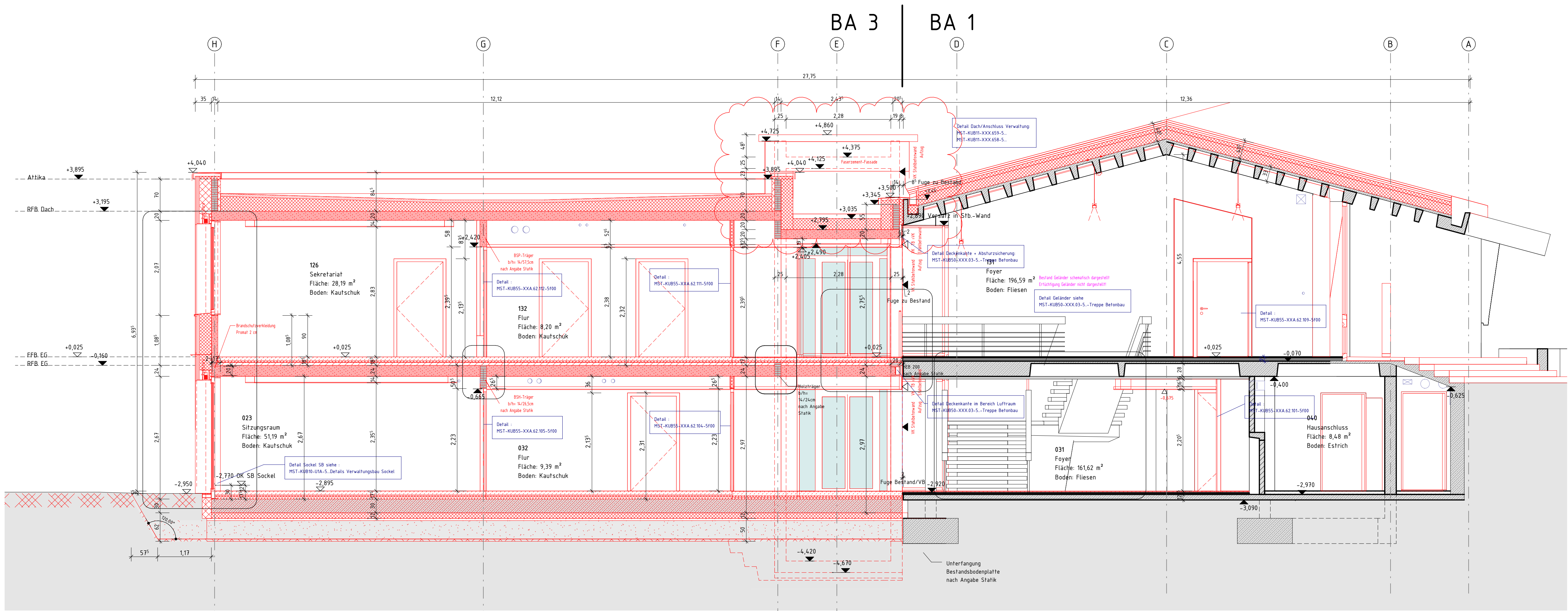
S03 - BA 3 M 1 : 50
